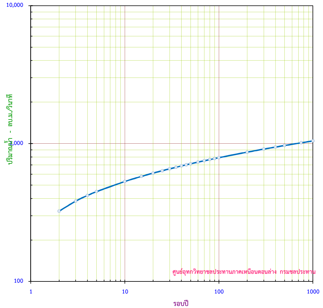
กราฟแสดง ปริมาณน้ำสูงสุดรายปี ขนาดรอบปีต่างๆ สถานี Y.4 อ.เมือง จ.สุโขทัย
